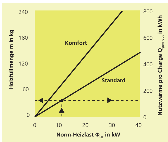
Auslegung Stückholzkessel
